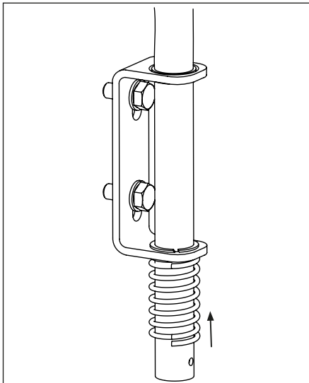
3. Feder montieren
