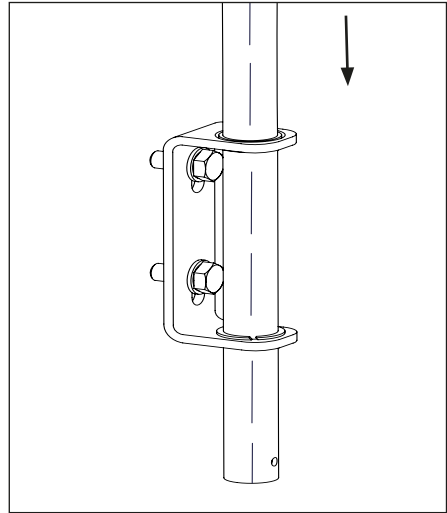
4. Spannhülse montieren
