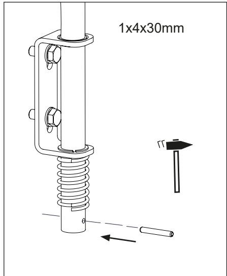
4. Spannhülse montieren
